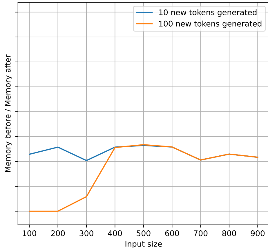
gpt2-xl
