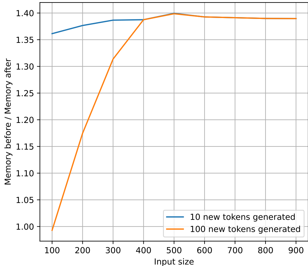
Bloom 7B
