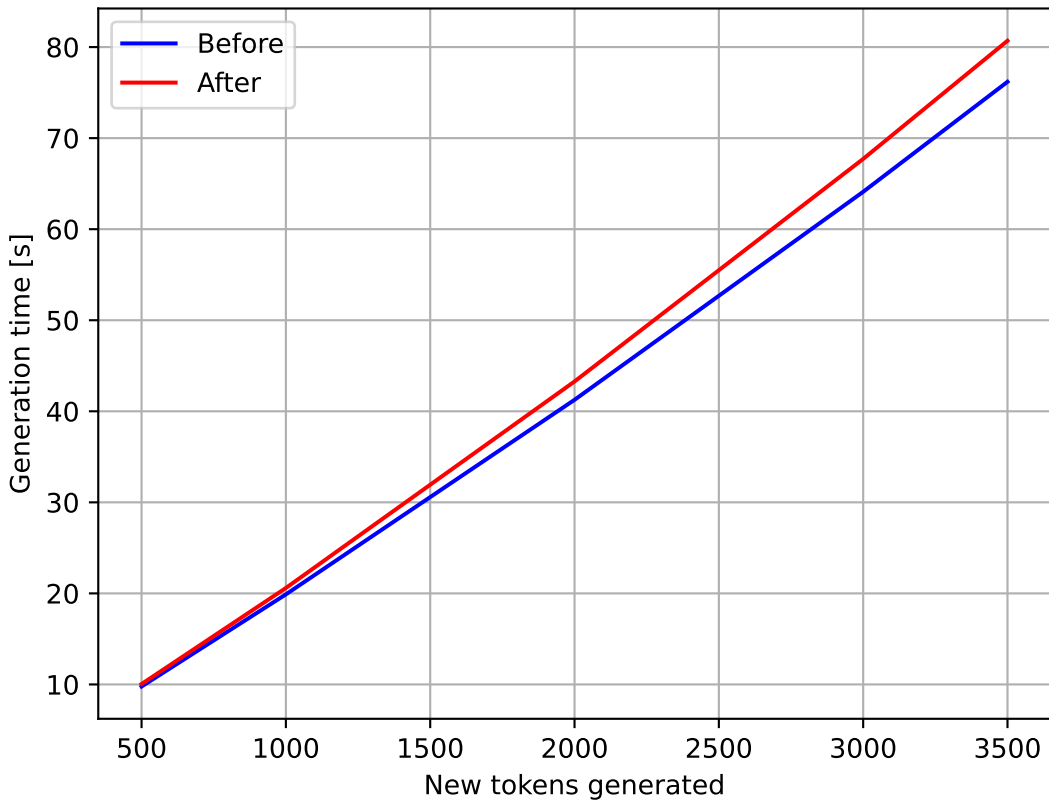
Llama-2-7b-hf Input size 300, Batch size 1
